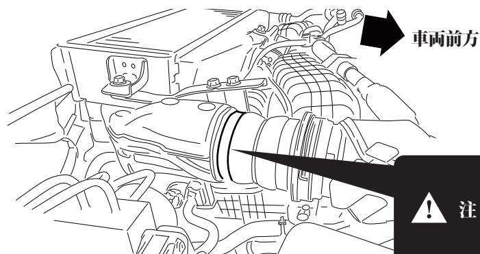
インタークーラーステーボルト/スロットルボディ部ボルト トルク 16Nm (1.6kgf-m)
