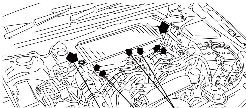
インタークーラーステーボルト/スロットルボディ部ボルト トルク 16Nm (1.6kgf-m)
